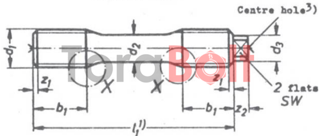
DIN 2510 Dimensions of Studs Metal End = 1xd
